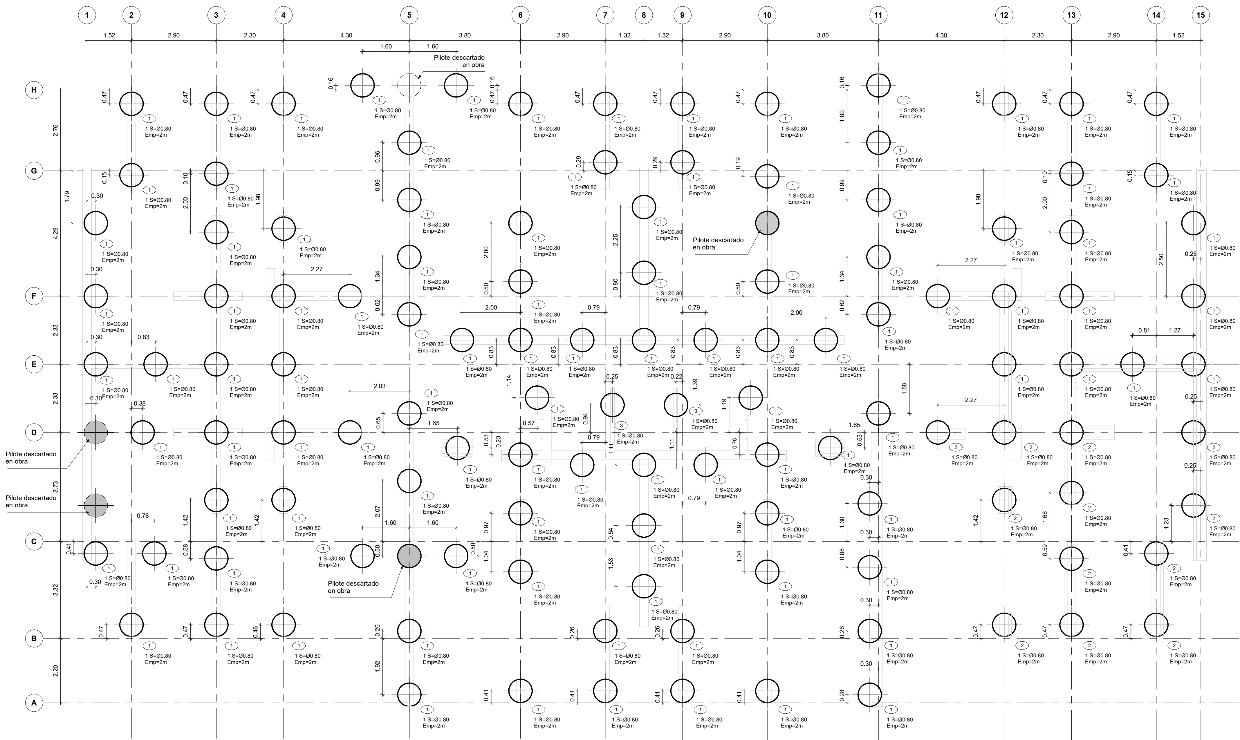
PLANTA DE LOCALIZACIÓN PILOTES Escala 1 : 75
